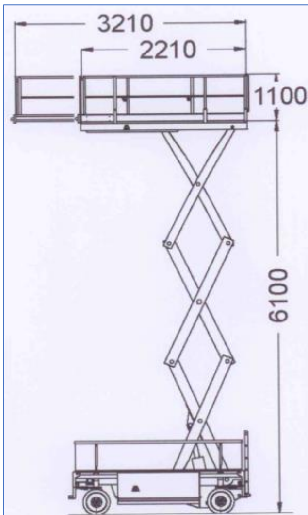
werkdiagram (Zijaanzicht)
